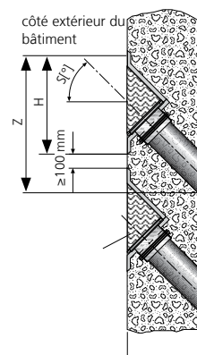
HSI150 1xZ KS45°/X garniture d'étanchéité biseautée simple face
